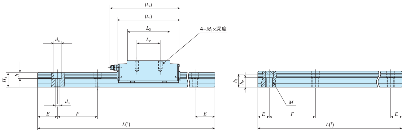
高密封滑轨下侧安装规格
