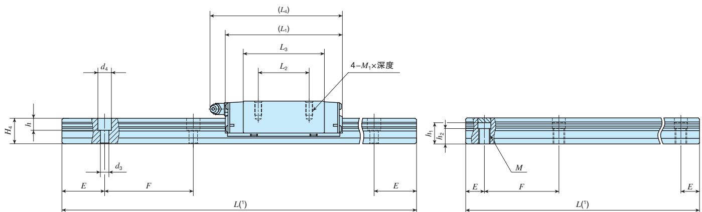
高密度滑轨下侧安装规格
