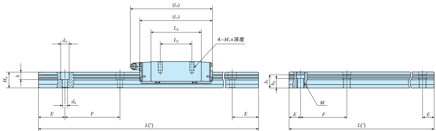
高密封滑轨下侧安装规格
