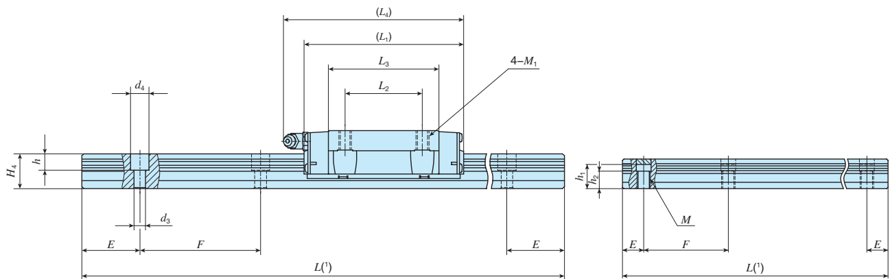
高密封滑轨下侧安装规格
