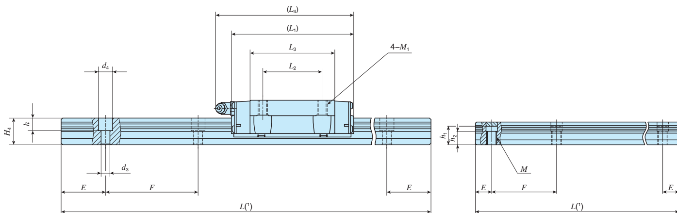
高密封滑轨下侧安装规格
